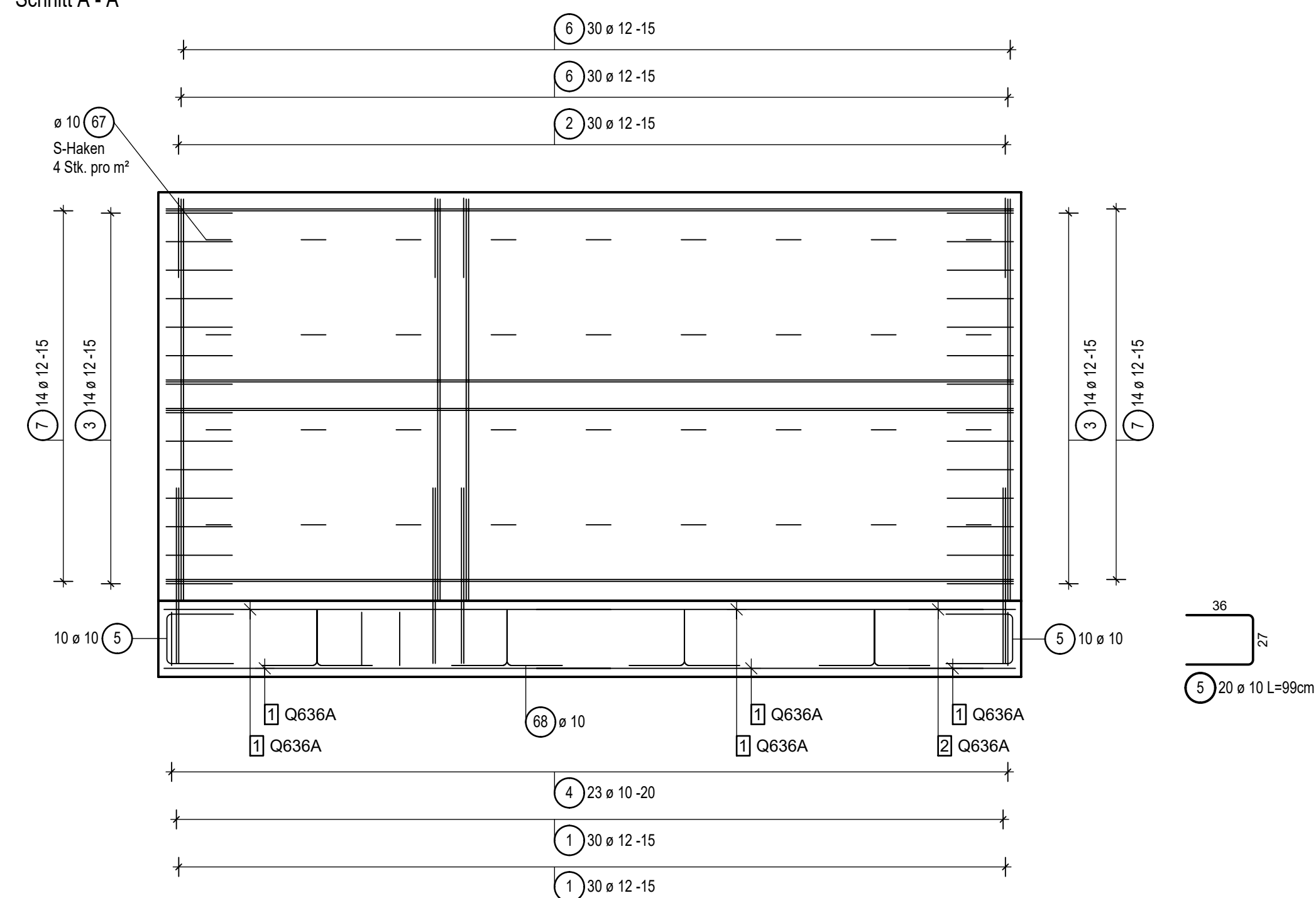
Schnitt A - A
